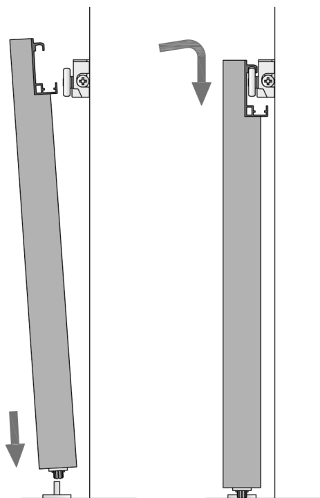
Установка двери
