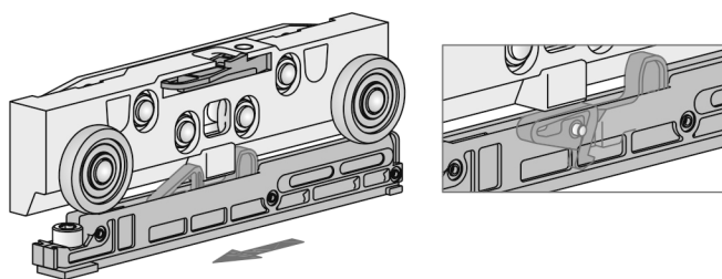
Доводчик
